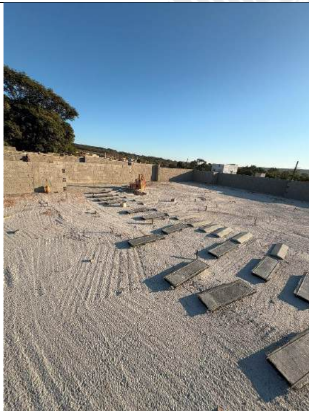
Foto 3 – Chapisco e execução de pingadeiras
