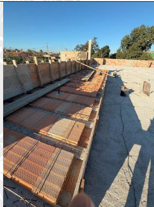
Foto 182 – Forma e concretagem de viga
