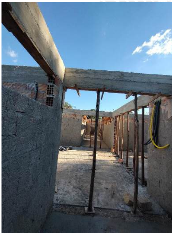
Foto 15 - Armação, forma e concretagem de cintas e vigas
