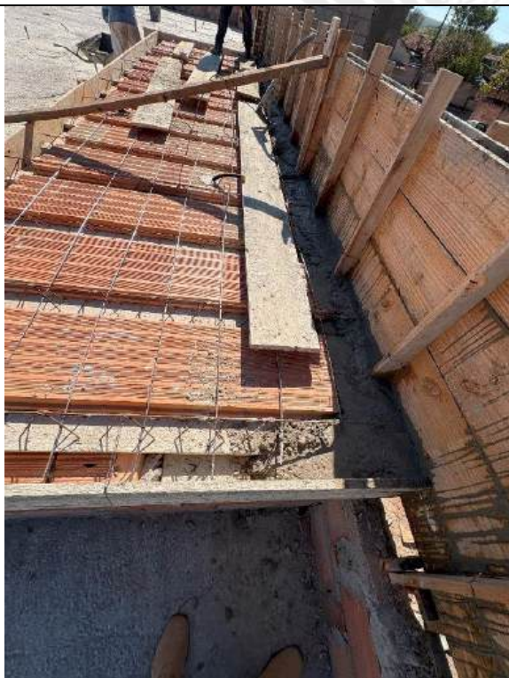
Foto 189 – Forma e concretagem de viga
