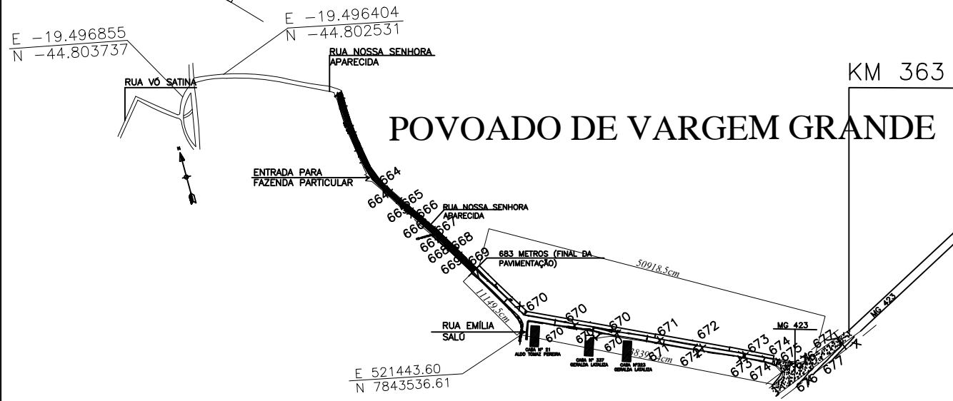
DETALHES PARA PAVIMENTAÇÃO SEM ESCALA
