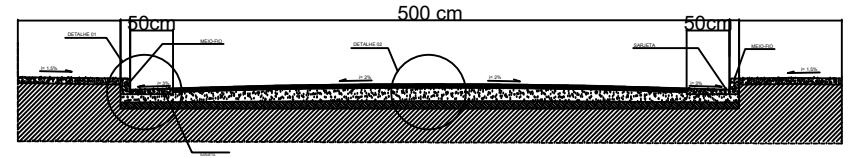
TRECHO 3 - RUA VÓ SATINA CORTE DA PISTA SEM ESCALA
