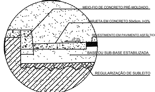
Detalhe 01
