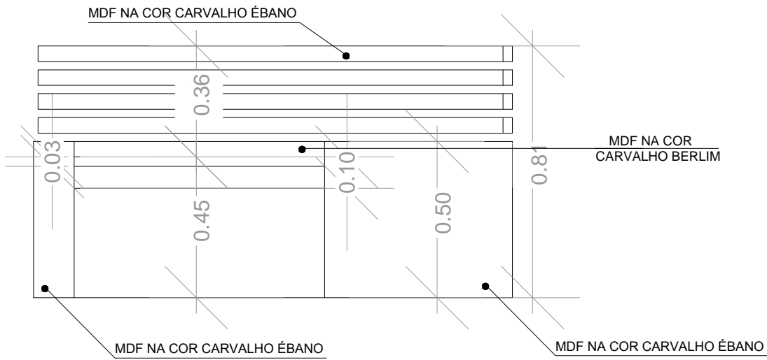
VISTA LATERAL DIREITA SOFÁ PEQUENO ESCALA: SEM ESCALA
